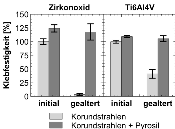
Relative Festigkeit an Zirkoniumdioxid und Titan (Ti6Al4V) mit Korundstrahlen oder Korundstrahlen + Pyrosil (Flampyolyse) als Oberflächenvorbehandlung infolge der hydrothermalen Alterung, jeweils normiert auf Korundstrahlen im Initialzustand (ohne Alterung)
